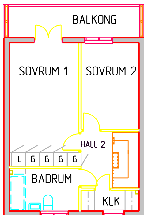
Övre plan
